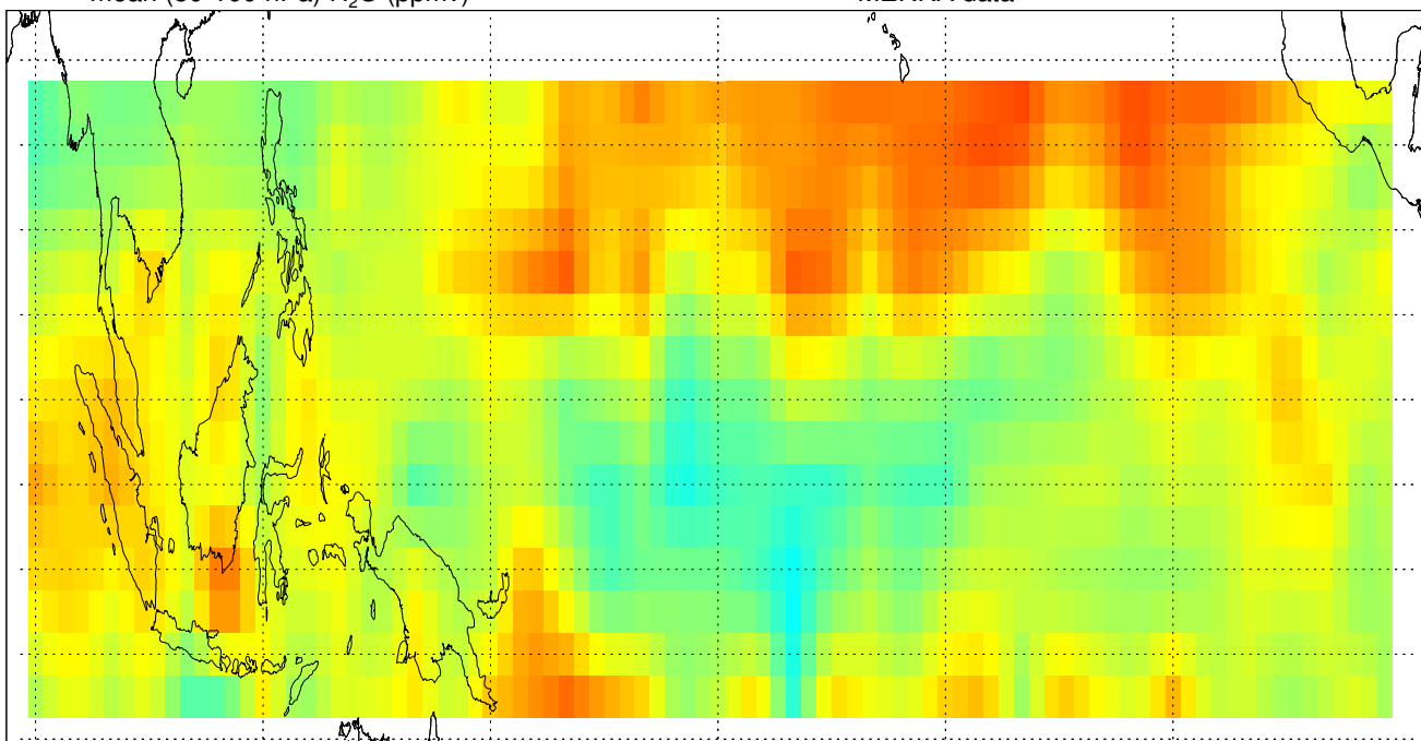
MERRA data
